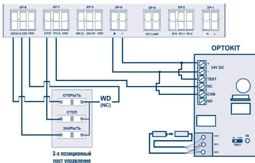
Рис. 1.2.2. Схема подключения трехпозиционного поста управления, датчика открытой калитки и оптосенсоров
