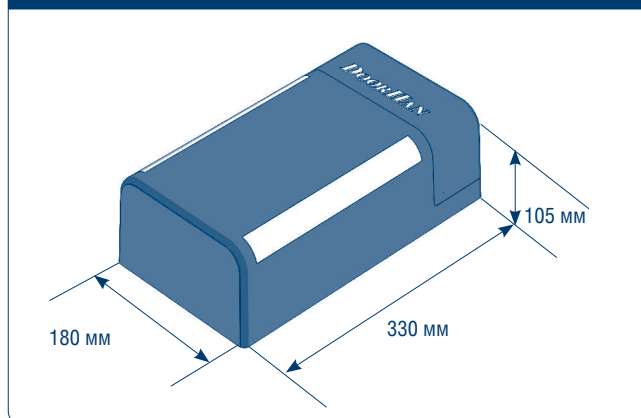
Рис. 1.2. Габаритные размеры
