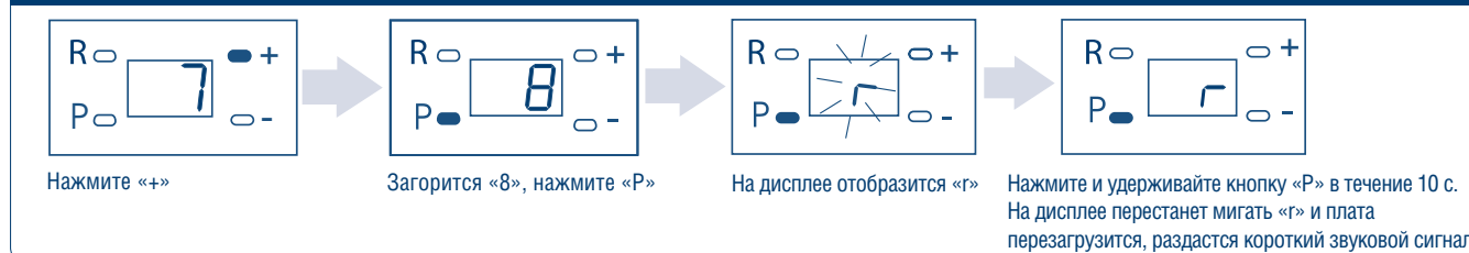
Рис. 6.3.8. Сброс параметров на заводские настройки
