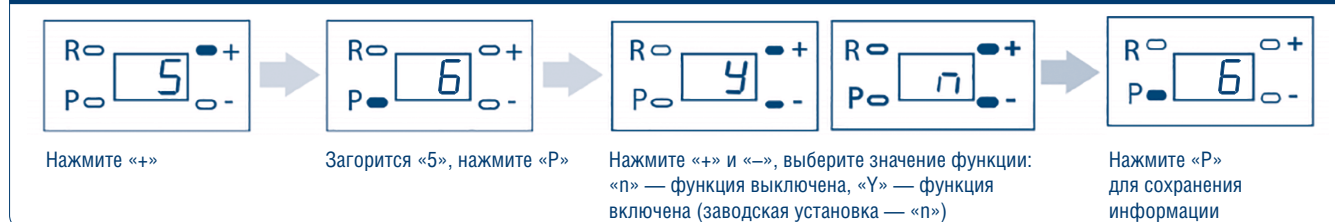
Рис. 6.3.6. Реверс каретки в закрытом положении ворот
