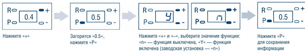
Рис. 6.4.6. Функция дистанционного управления дополнительным внешним освещением
