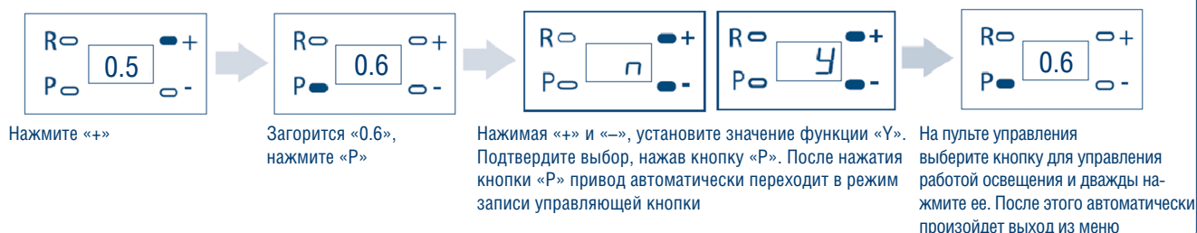
Рис. 6.4.6. Функция дистанционного управления дополнительным внешним освещением
