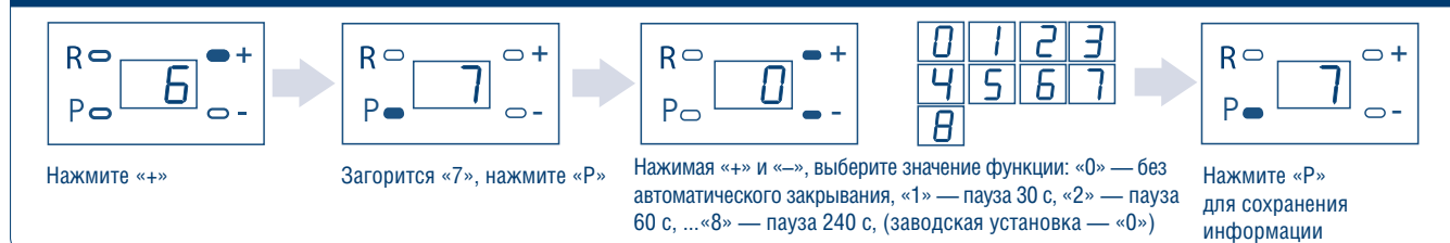
Рис. 6.3.7. Автоматическое закрывание открытых ворот
